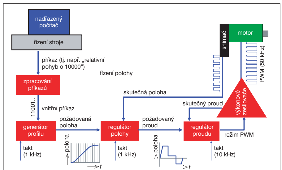
Obr. 2. Uspořádání řídicí jednotky EPOS
