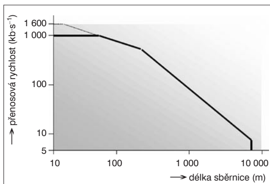
Obr. 5. Vliv délky sběrnice CAN na přenosovou rychlost
