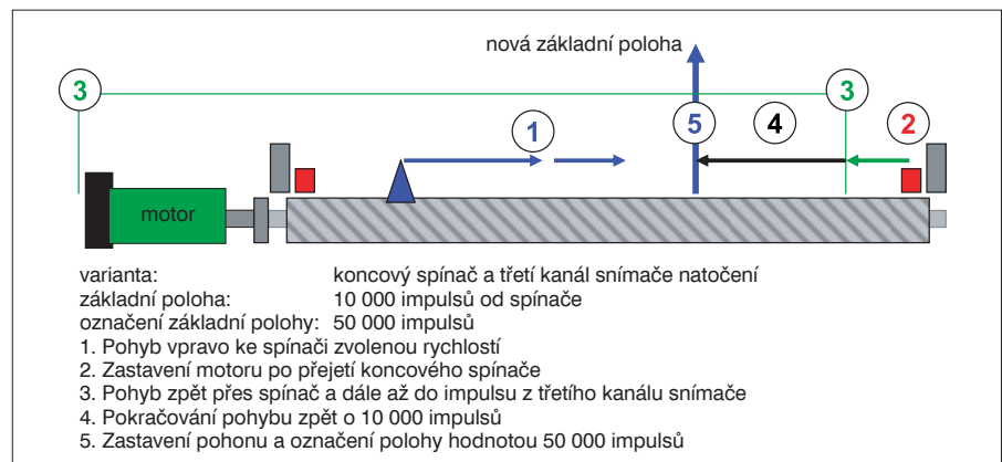
Obr. 4. Nastavení základní polohy pohonu
